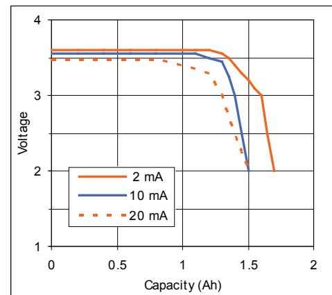
150°C discharge
